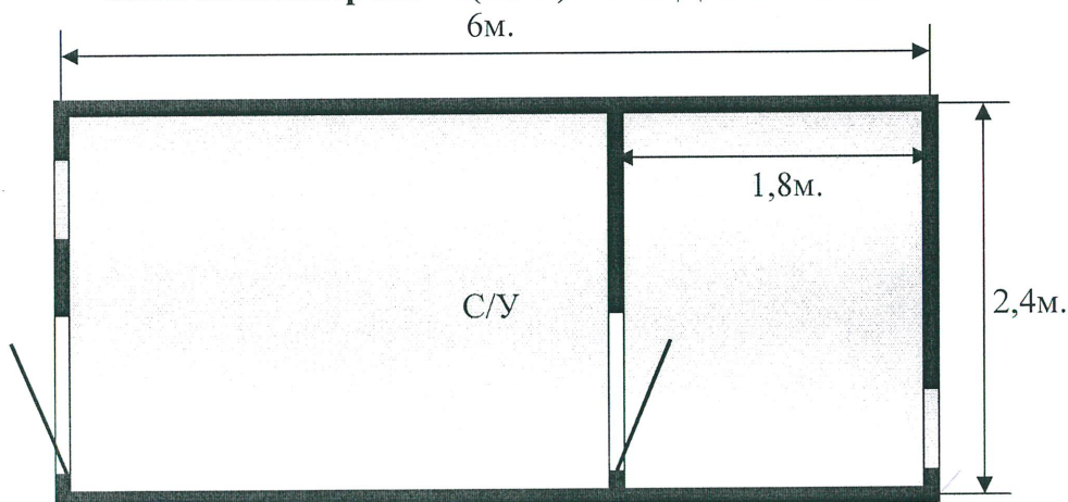
Блок-контейнер БК-03(ПВХ) СТАНДАРТ – 1шт.
