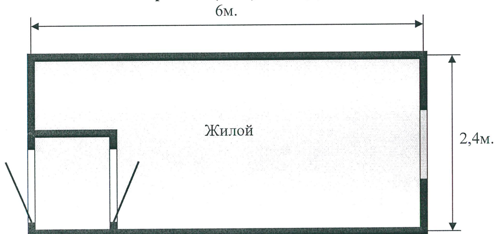
Блок-контейнер БК-01(ВАГ) СТАНДАРТ – 11шт.
